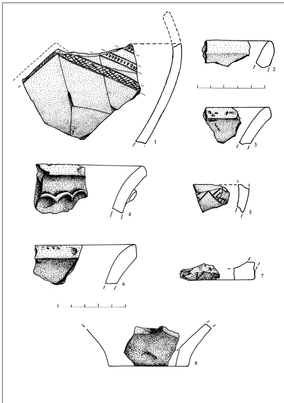
Pl. 1. Ceramică aparținând culturii Wietenberg de la Meteș – Vârful Băii
